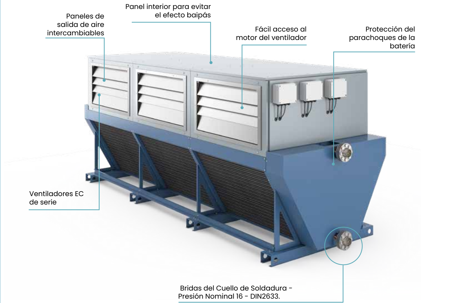
Panel interior para evitar el efecto baipás
